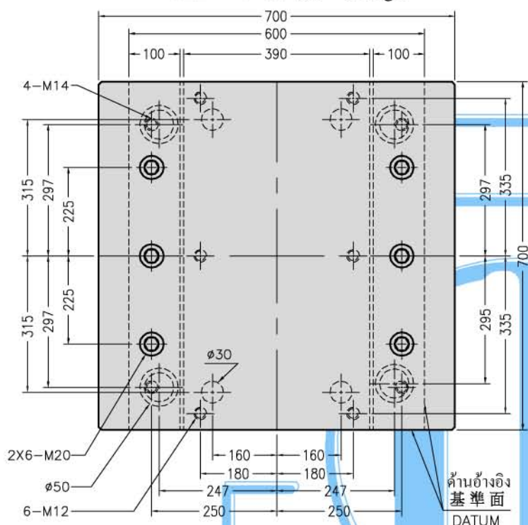
แบบ 平面圖 Design
