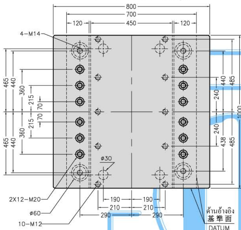
แบบ 平面圖 Design
