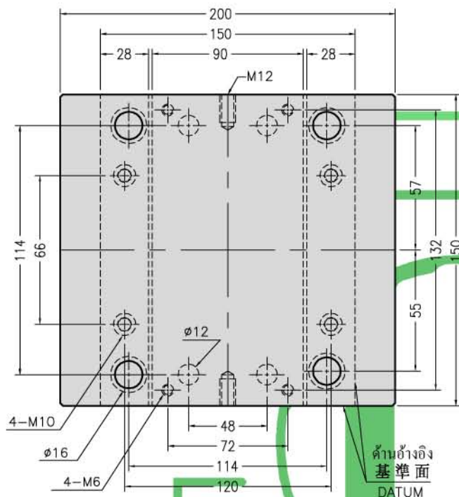
แบบ 平面圖 Design
