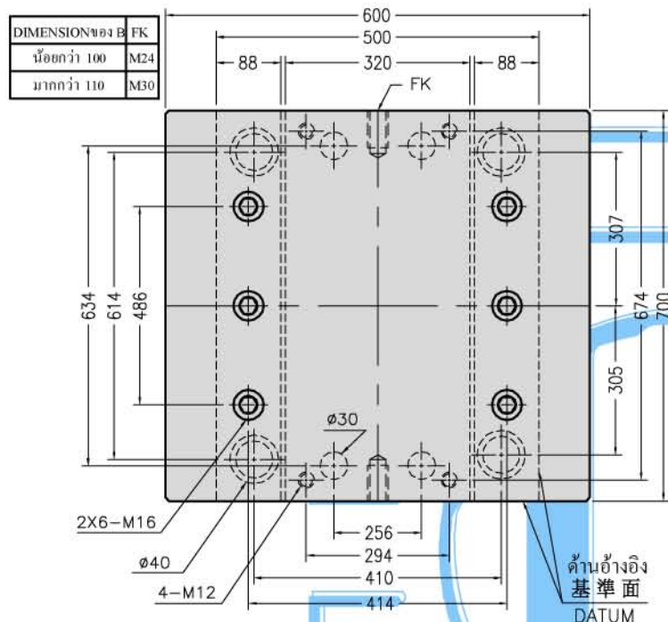
แบบ 平面圖 Design
