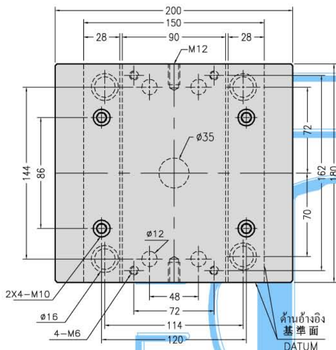
11.1 平面圖 Design
