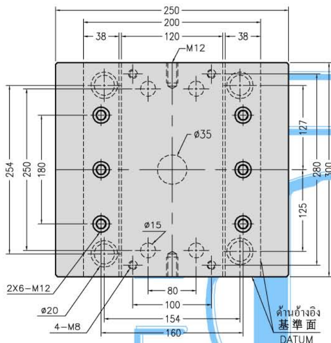
၈၈၈ 平 面 圖 Design
