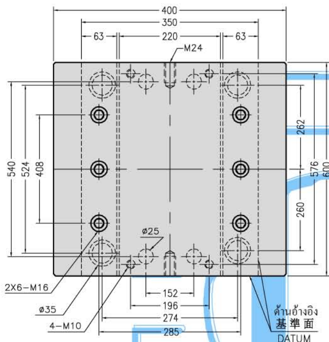
แบบ 平面圖 Design
